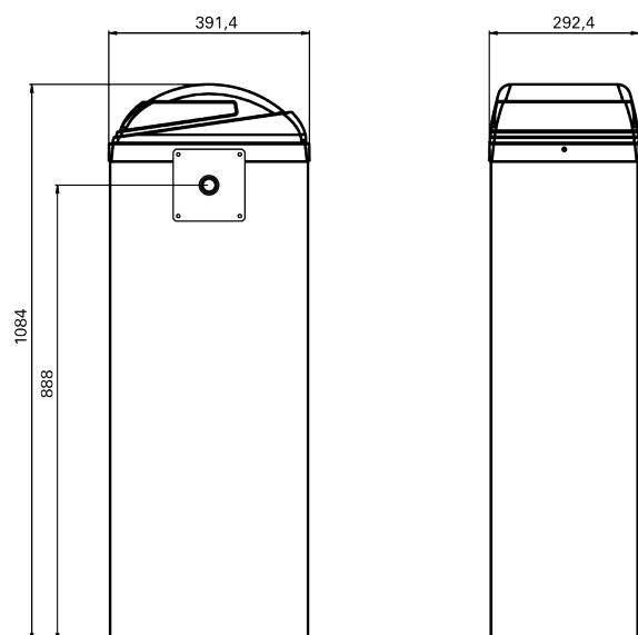
DIMENSIONS DE LA BARRIERE
